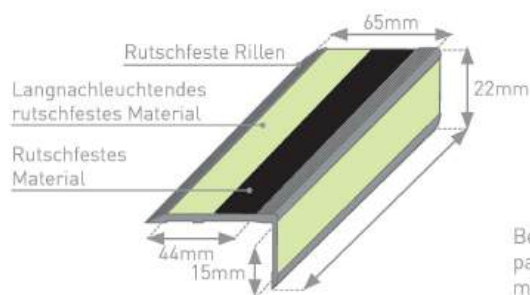
Trappebeskyttelse
